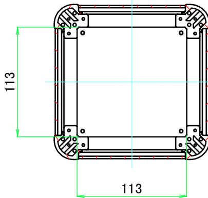
C-C ( 1 : 4 )
